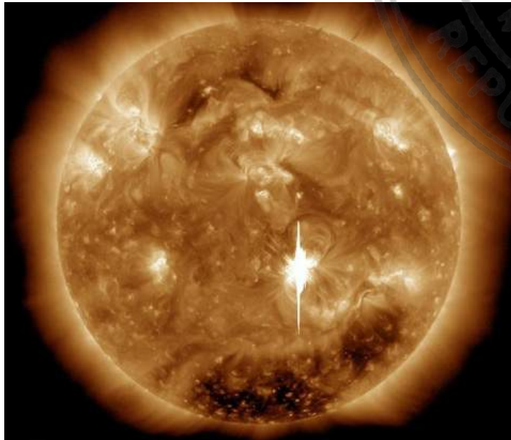
Gambar 24. Matahari dilihat dengan teleskop.
