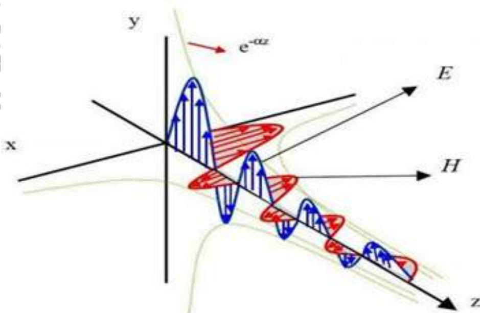
Gambar 12. Cahaya sebagai Gelombang Elektromagnetik.
