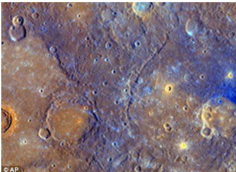
Gambar 44. Planer Merkurius sangat panas dan tak ada perlindungan atmosfer sehingga sering mengalami tumbukan meteorit yang membuatnya penuh kawah. (Dari http://www.dailymail.co.uk/sciencetech/article-1081833/Smallest-planet-Mercury-volcanic-activity-say-NASA-space-scientists.html )
