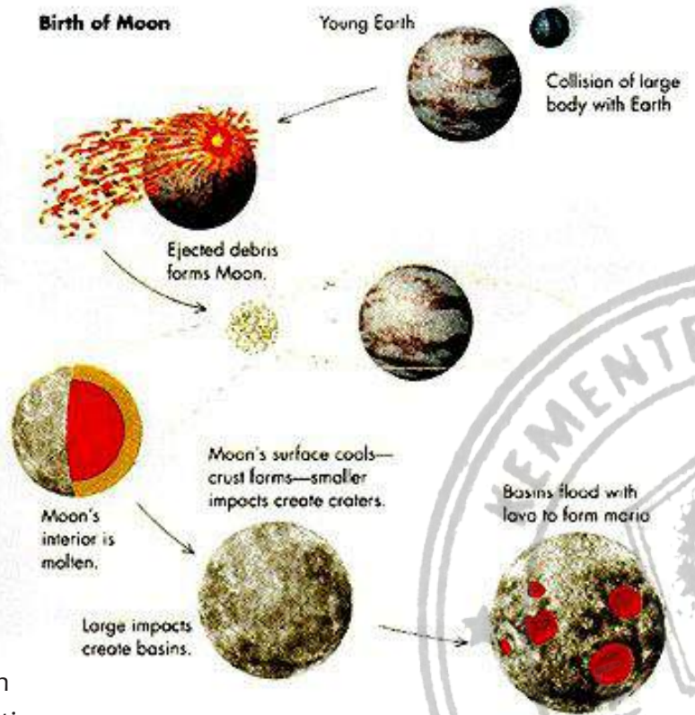
Gambar 36. Asal usul bulan diteorikan berasal dari bumi juga. (dari http://www.solarsystem.ie/images/full-birth_of_moon.jpg )
