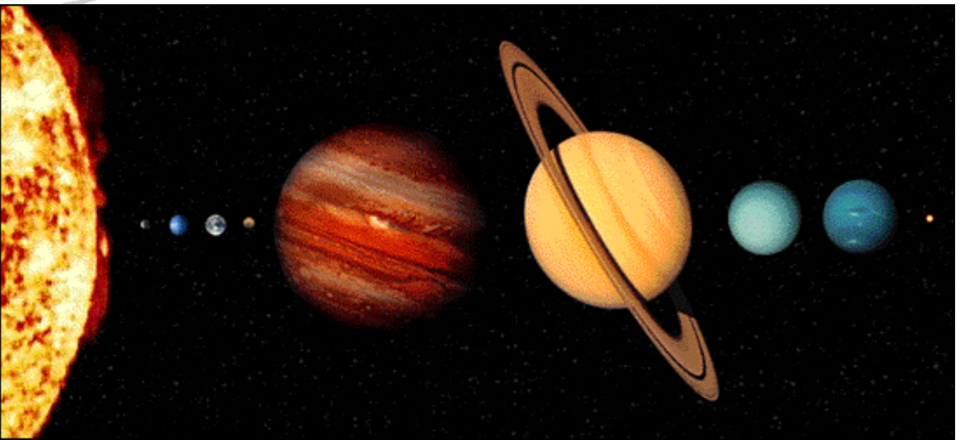
Gambar 43. Tata surya terdiri empat planet kecil keluarga bumi dan empat planet raksasa keluarga Jupiter. (Dari http://coolcosmos.ipac.caltech.edu/ )
