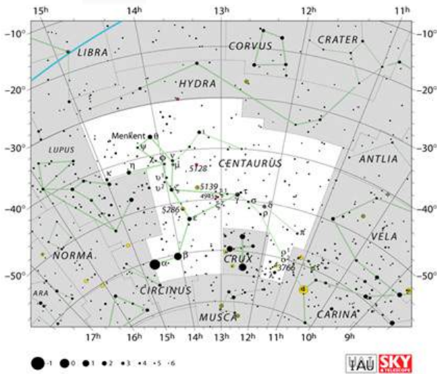
Gambar 2. Peta rasi Centaurus, lokasi bintang Alfa dan Beta Centauri berada.
