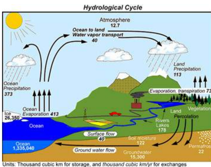
Gambar 27. Matahari sebagai penggerak cuaca dan siklus hidrologi. (Dari http://www.tiimes.ucar.edu/highlights/fyo6/dai.html )
