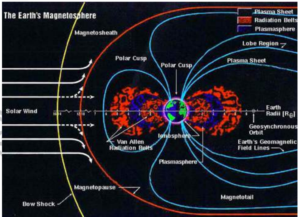
Gambar 18. Medan magnet bumi dan sabuk van Allen
