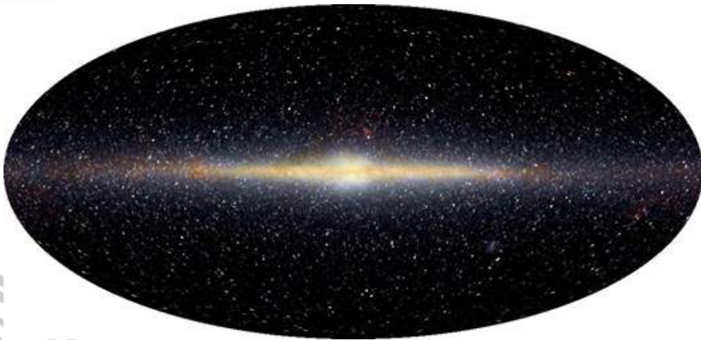
Gambar 4. Distribusi objek inframerah yang direkam satelit COBE dalam galaksi kita, Galaksi Bimasakti.
