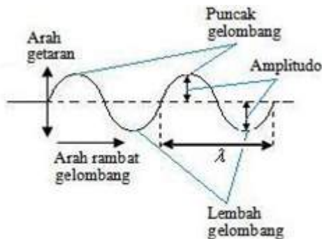
Gelombang transversal
