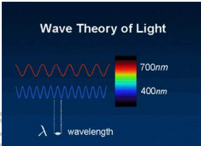
Gambar 11. Teori gelombang cahaya.
