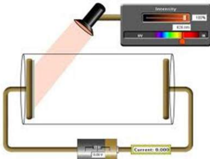
Gambar 15. Efek Fotolistrik
