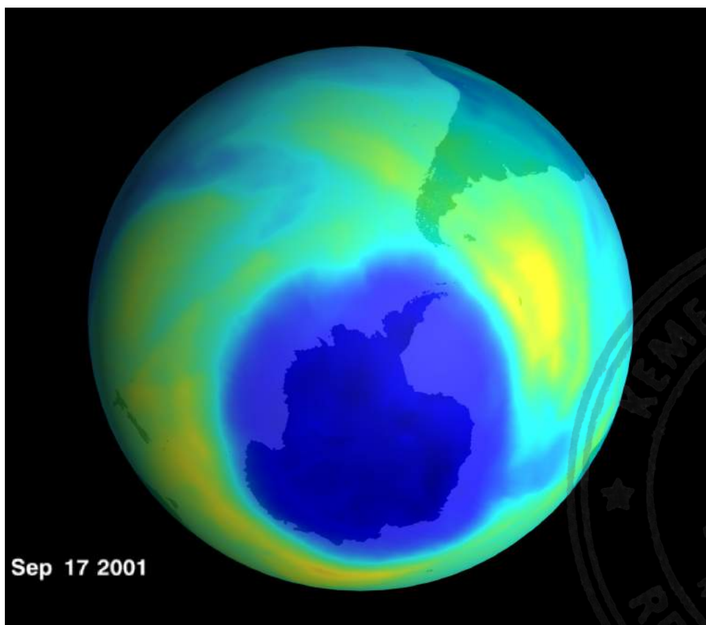
Gambar 7. Lubang ozon makin luas di Antartika akibat ulah manusia. Sumber: earthobservatory.nasa.gov
